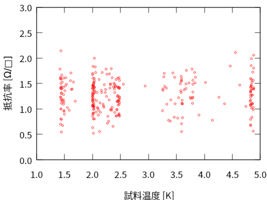
図2 Si(111)-(7×7)表面上にスズを蒸着して作製した Si(111)-( \sqrt{3} \times \sqrt{3} )-Sn 試料の抵抗率の温度依存性。1.4 K から 5.0 K の温度で 1.3 Ω/□ 程度とほぼ一定の値を示した。
