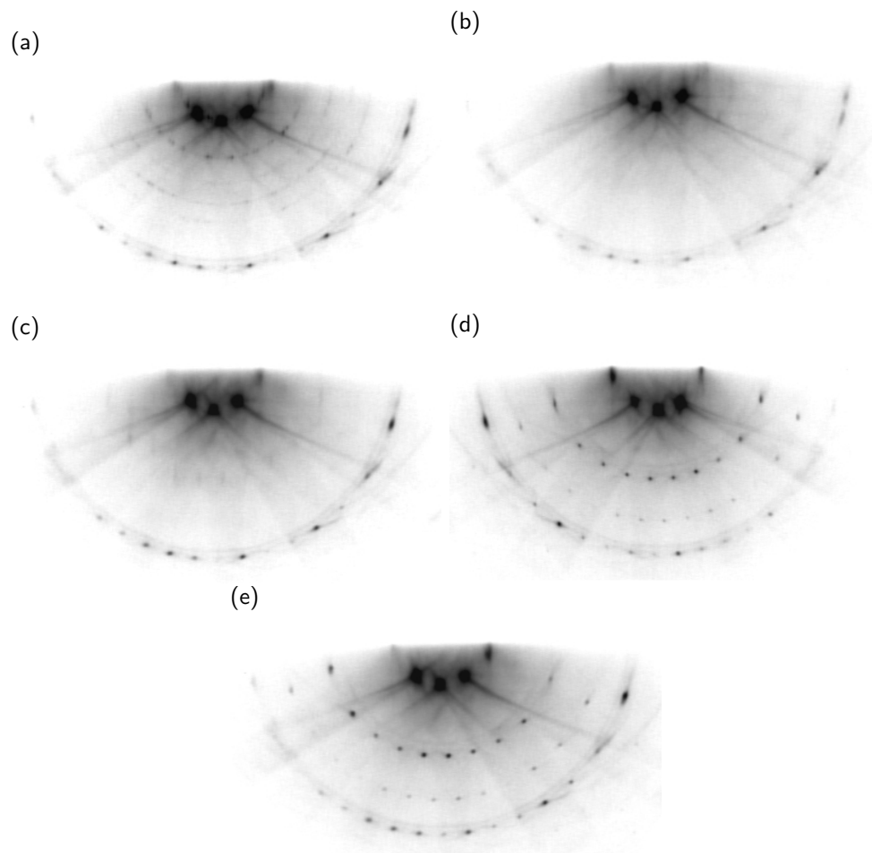
図 1 (a) 基板の表面を清浄化して得られた Si(111)- 7 \times 7 表面の RHEED パターン。(b, c) 基板を約 1250^\circ\text{C} に加熱する操作を繰り返すと表面にドーパントのホウ素が偏析して (b) のように 7 \times 7 のスポットが見えなくなり、さらに同様の操作を続けることによって (c) のように \sqrt{3} \times \sqrt{3} -B 構造ができる。(d) 基板を約 600^\circ\text{C} に保ちながら Si(111)- 7 \times 7 表面上にスズを 1/3 原子層蒸着することによって Si(111)-( \sqrt{3} \times \sqrt{3} )-Sn が得られる。(e) 表面にホウ素が偏析して (c) のようになった基板上でも (d) と同様にスズを蒸着することによって Si(111)-( \sqrt{3} \times \sqrt{3} )-Sn が得られる。なお、(b) のような表面の基板についても、スズの蒸着によって同様の RHEED パターンが得られた。(a-e) いずれも電子線の入射方向は \langle \bar{1}10 \rangle である。
